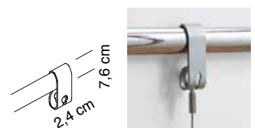
5166-GA, 5166-BO
